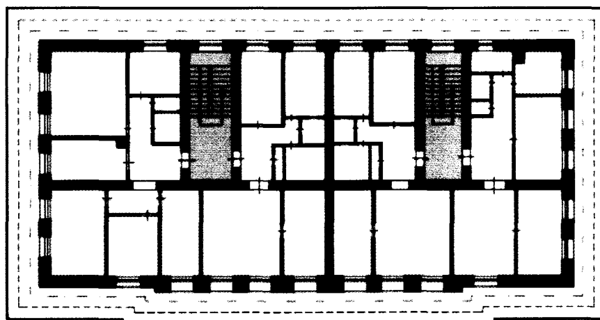
План 3 этажа
