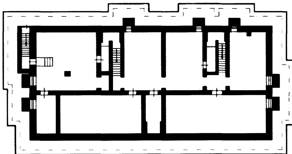
План подвала
