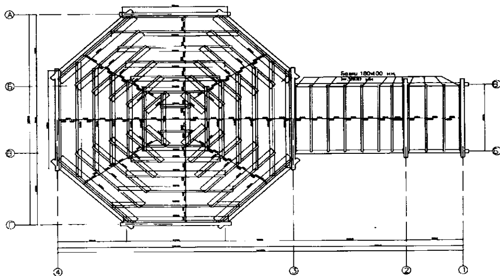
ПЛАН ПЕРЕКРЫТИЯ М1:100
