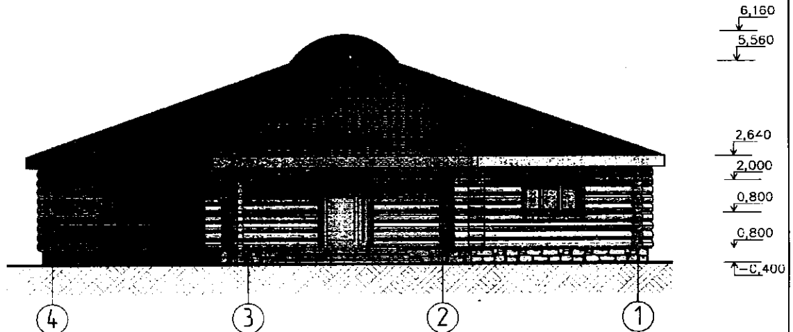
Фасад по осям 4-1
