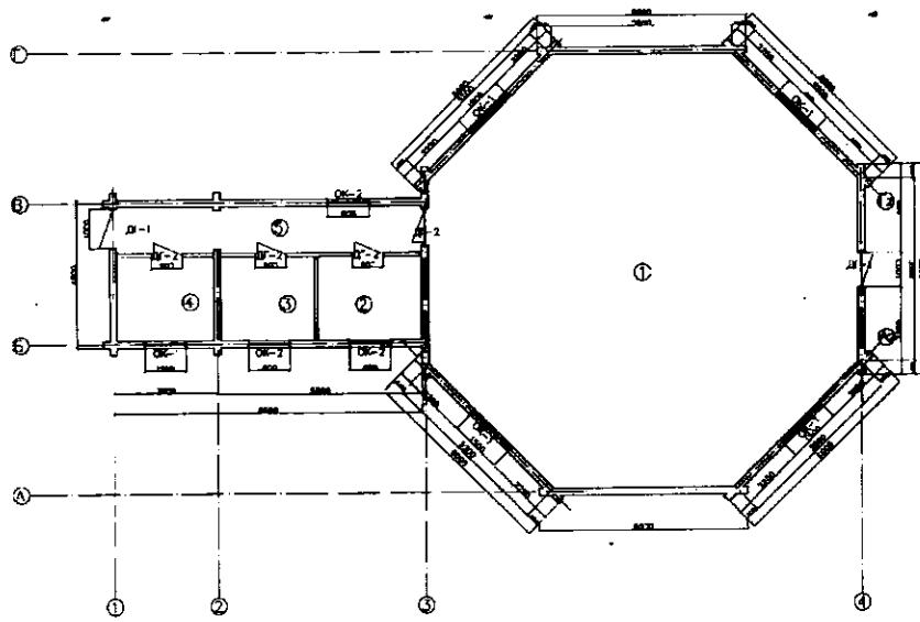
ПЛАН ЗДАНИЯ М1:100
