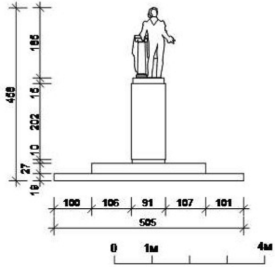
Обмеры 25.06.1980 г.
