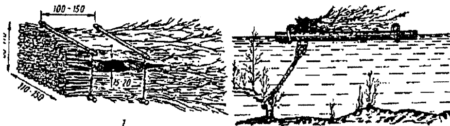
Рисунок 63. Варианты сооружений для спасения пушных животных в половодье (по Харченко, 2005)
