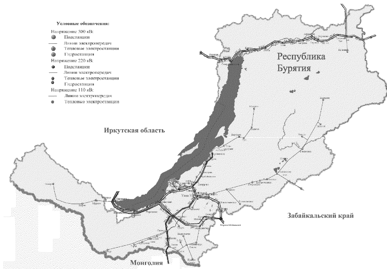
Рисунок 9.1-1. Карта-схема электрических сетей Республики Бурятия
