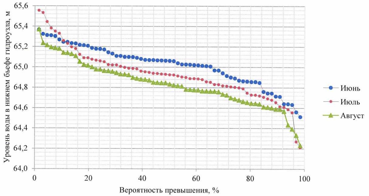
Кривые продолжительности конечных для интервала уровней воды в нижнем бьефе гидроузла Камбарского водохранилища (июнь – август)
