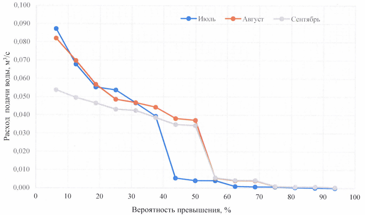
Кривые продолжительности средних за интервал расходов подачи воды участникам водохозяйственного комплекса в Камбарском водохранилище (июль – сентябрь)
