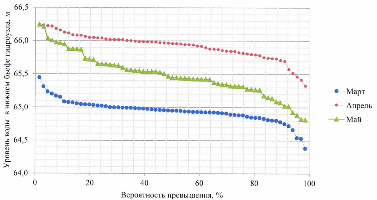
Кривые продолжительности конечных для интервала уровней воды в нижнем бьефе гидроузла Камбарского водохранилища (март – май)
