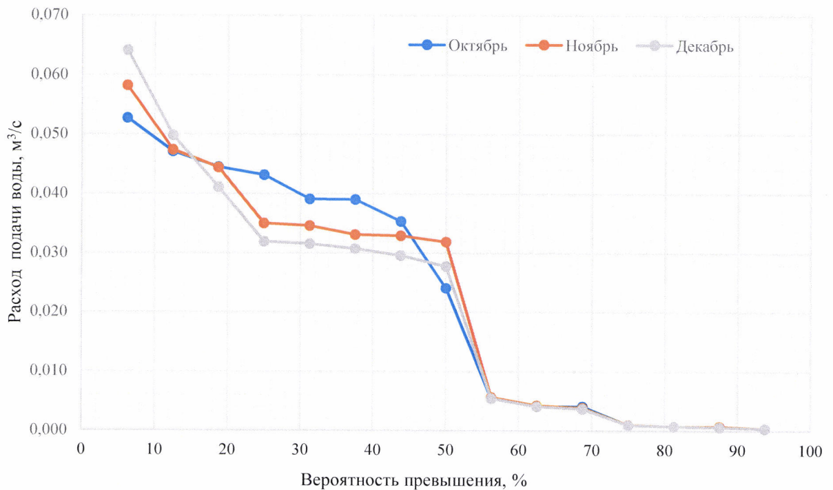
Кривые продолжительности средних за интервал расходов подачи воды участникам водохозяйственного комплекса в Камбарском водохранилище (октябрь – декабрь)
