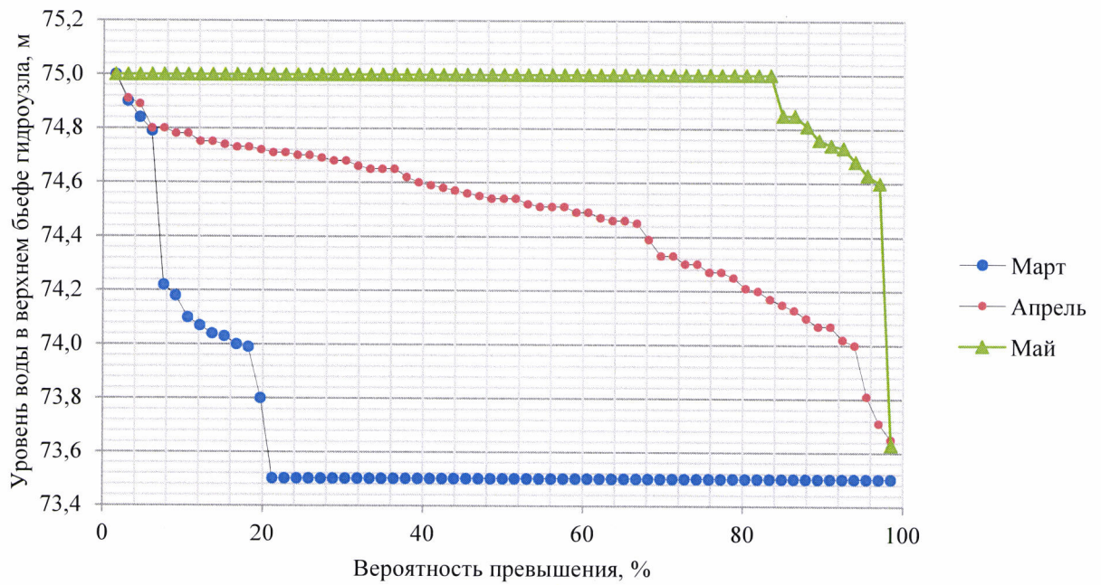
Кривые продолжительности конечных для интервала уровней воды в Камбарском водохранилище (март – май)
