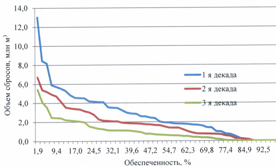
Расчетная обеспеченность объемов сбросов в нижний бьеф гидроузла Приморского водохранилища за первую декаду мая
