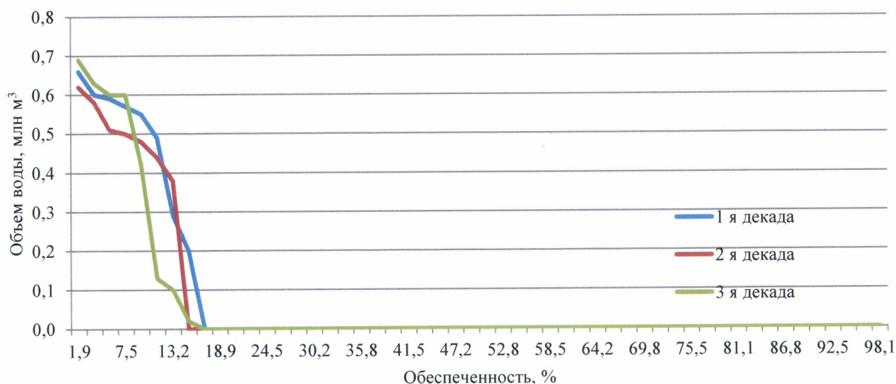
Расчетная обеспеченность объемов подпитки Приморского водохранилища за первую декаду октября
