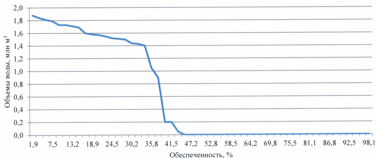
Расчетная обеспеченность объемов подпитки Приморского водохранилища Расчетная обеспеченность объемов подпитки Приморского водохранилища за январь
