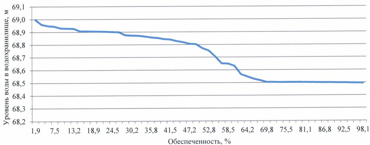
Расчетная обеспеченность уровней Приморского водохранилища за декабрь
