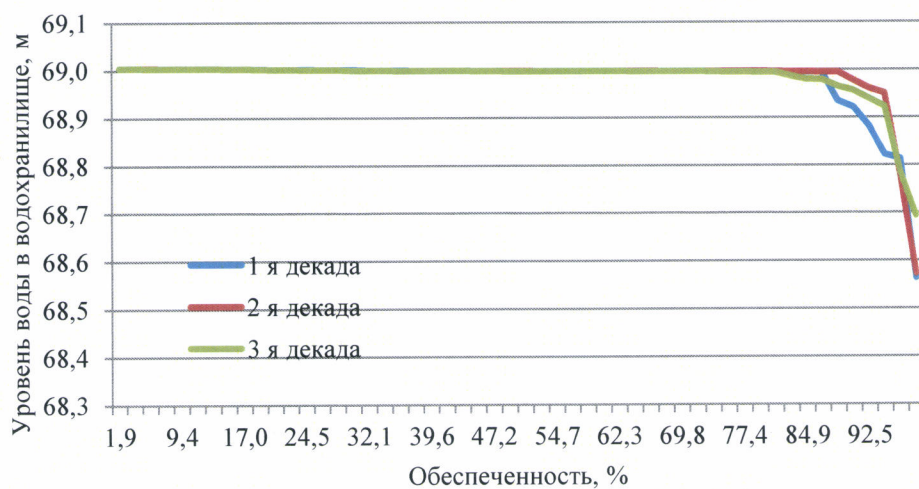
Расчетная обеспеченность уровней Приморского водохранилища за первую декаду мая
