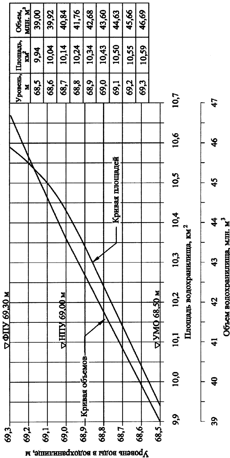
Статические кривые зависимости объемов воды и площадей зеркала Приморского водохранилища от уровней воды
