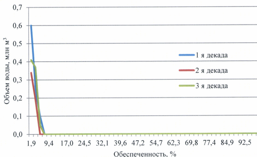
Расчетная обеспеченность объемов подпитки Приморского водохранилища за август
