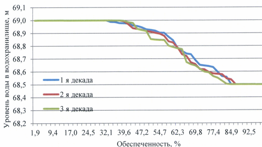
Расчетная обеспеченность уровней Приморского водохранилища за октябрь
