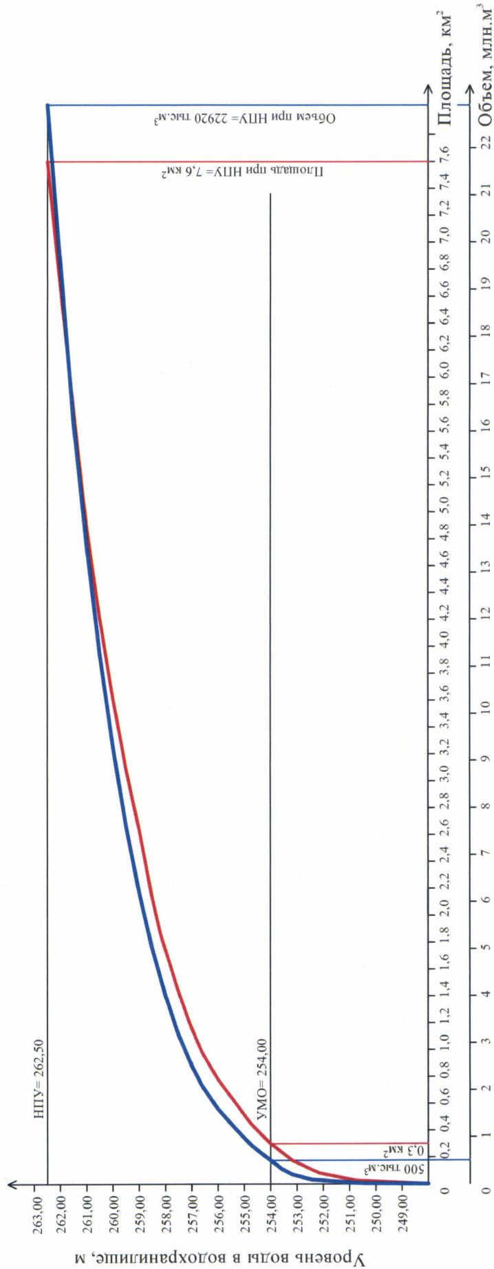
Статические кривые зависимости объемов воды и площадей зеркала Катенинского водохранилища от уровней воды
