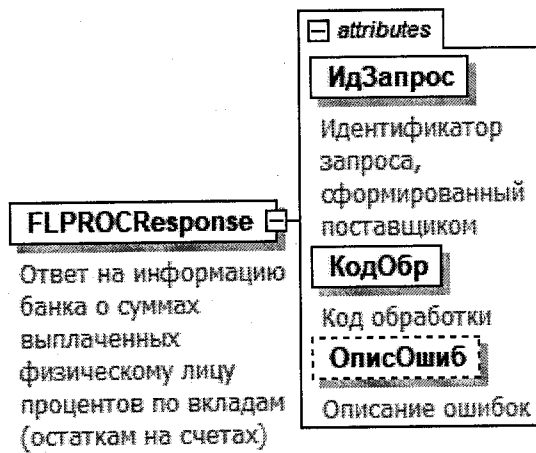
Рисунок 2. Диаграмма структуры файла обмена
