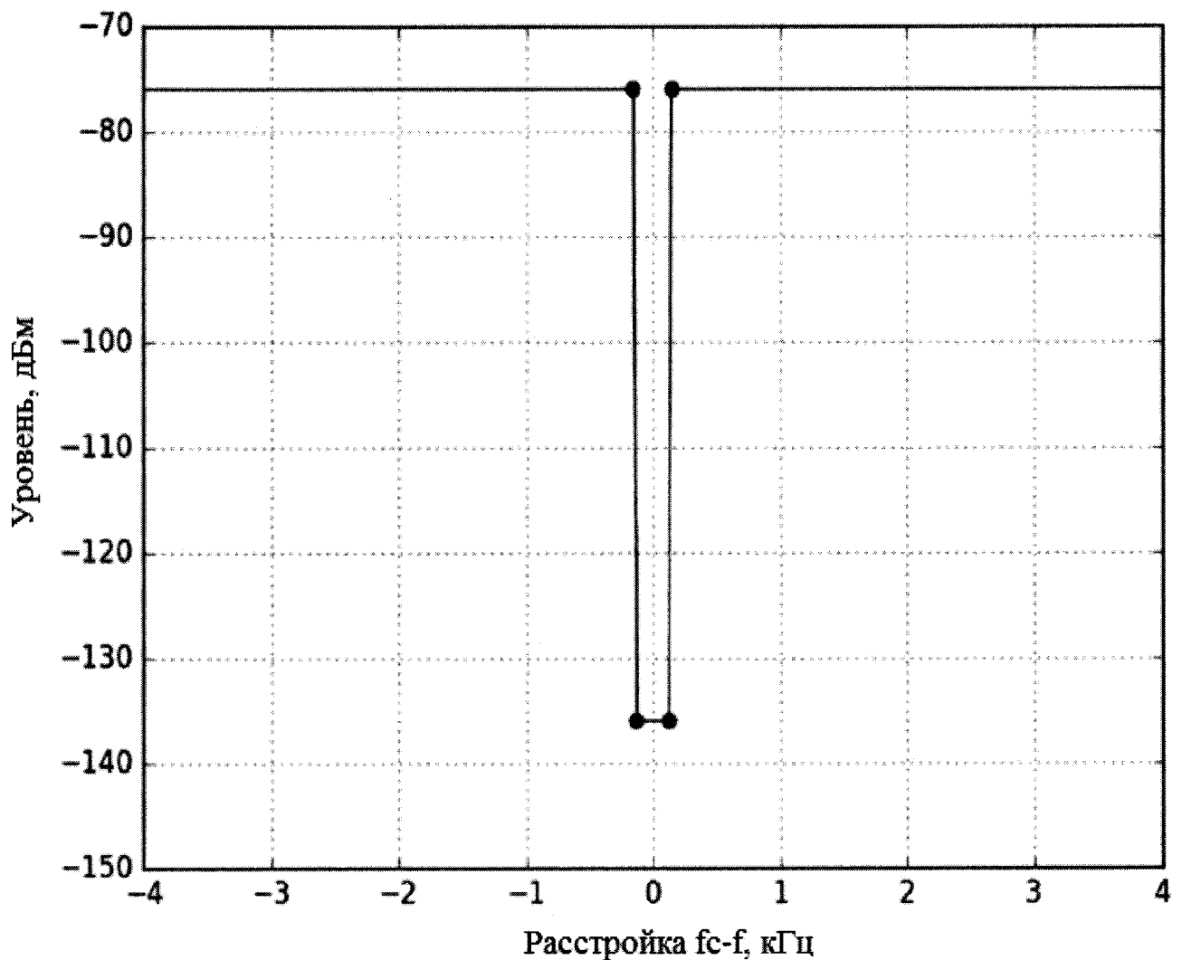
Рисунок 3. Маска уровней блокировки приемника для восходящей линии
