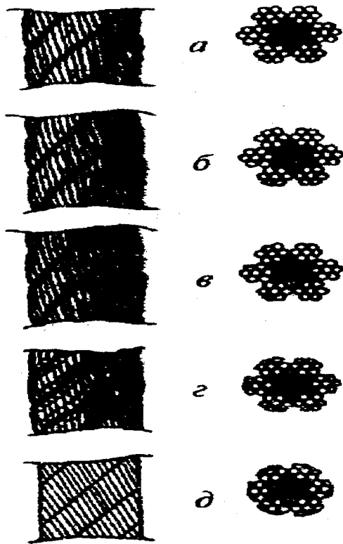
Рисунок 5. Износ наружных проволок каната крестовой свивки:
