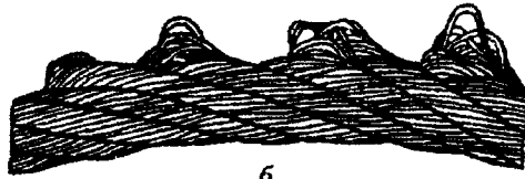
Рисунок 12. Выдавливание проволок прядей:
