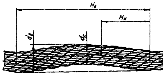
Рисунок 9. Волнистость каната
