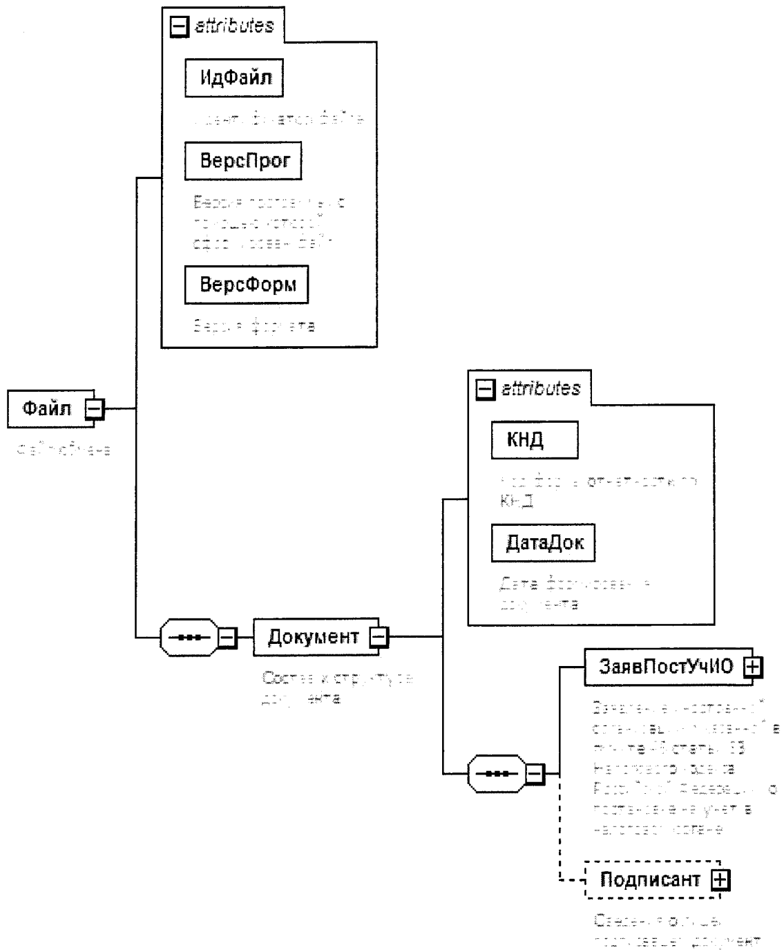
Рисунок 1. Диаграмма структуры файла обмена
