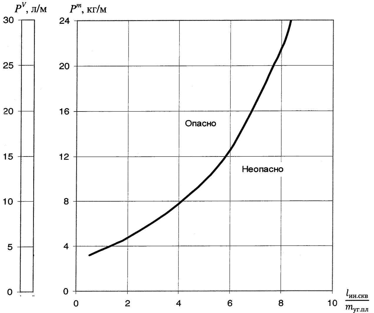
Рис. 1. Номограмма для установления категории «опасно» или «неопасно» участков каменноугольных пластов по выходу буровой мелочи:
