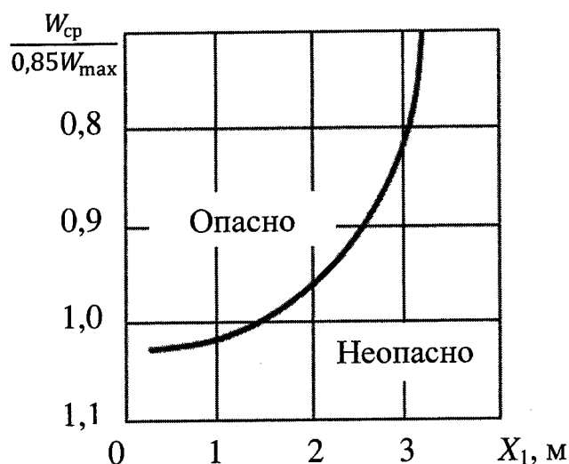
Рис. 4. Номограмма для установления категории «опасно» или «неопасно» участков бурогольных пластов по естественной влаге:
