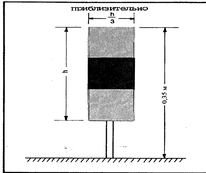
Рис. 10. Маркер РД для руления по воздуху
