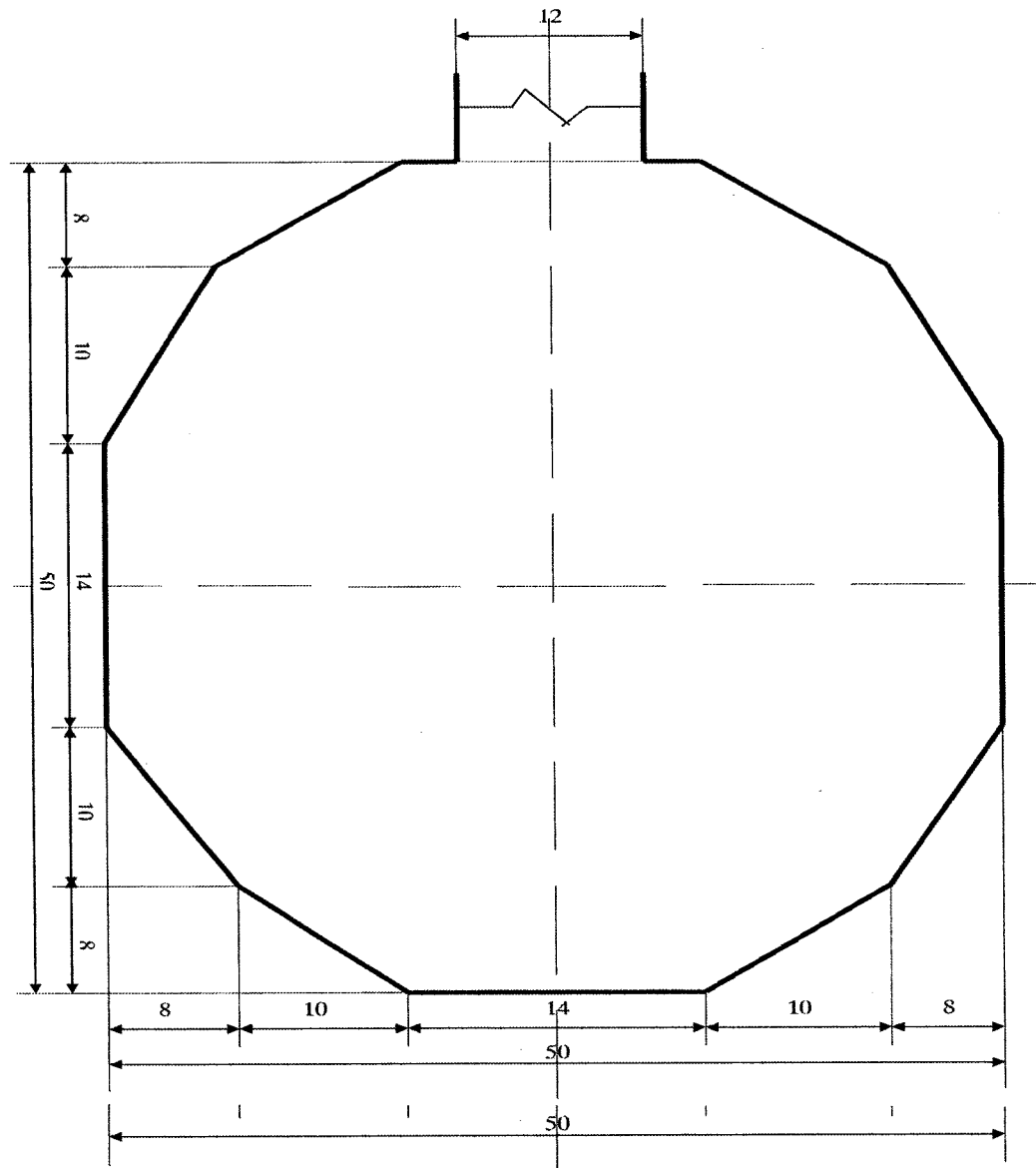
Рис. 4 Рекомендуемые размеры и конфигурация мест опробования силовых установок и девиационных площадок тяжелых и средних вертолетов
