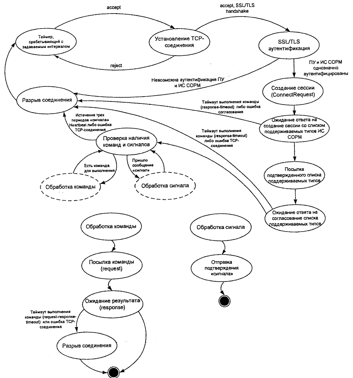
Рисунок 1. Диаграмма состояний перехода ПУ по кпд 1.
