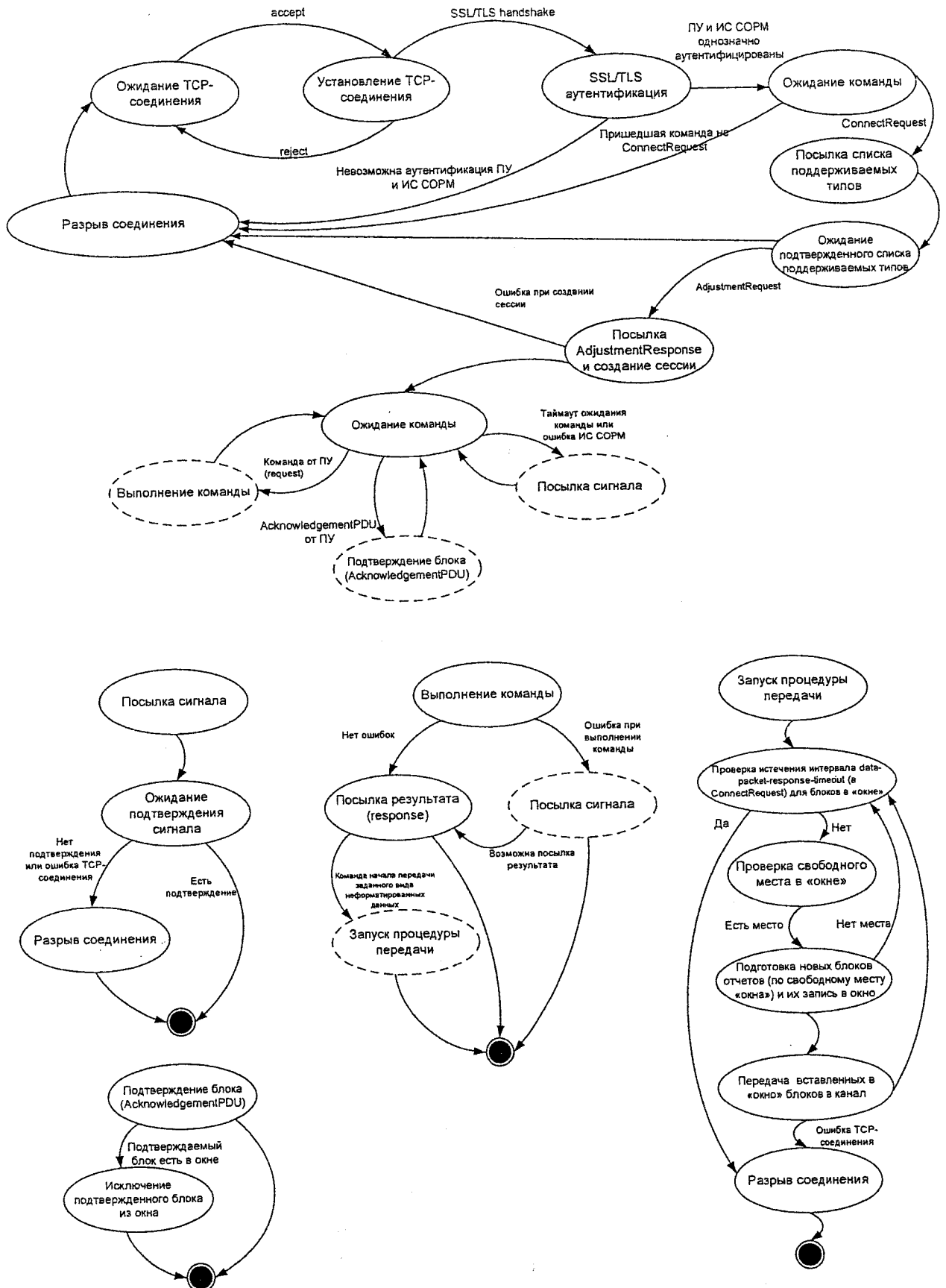
Рисунок 1. Диаграмма состояний перехода TC ORP по кпд 4.
