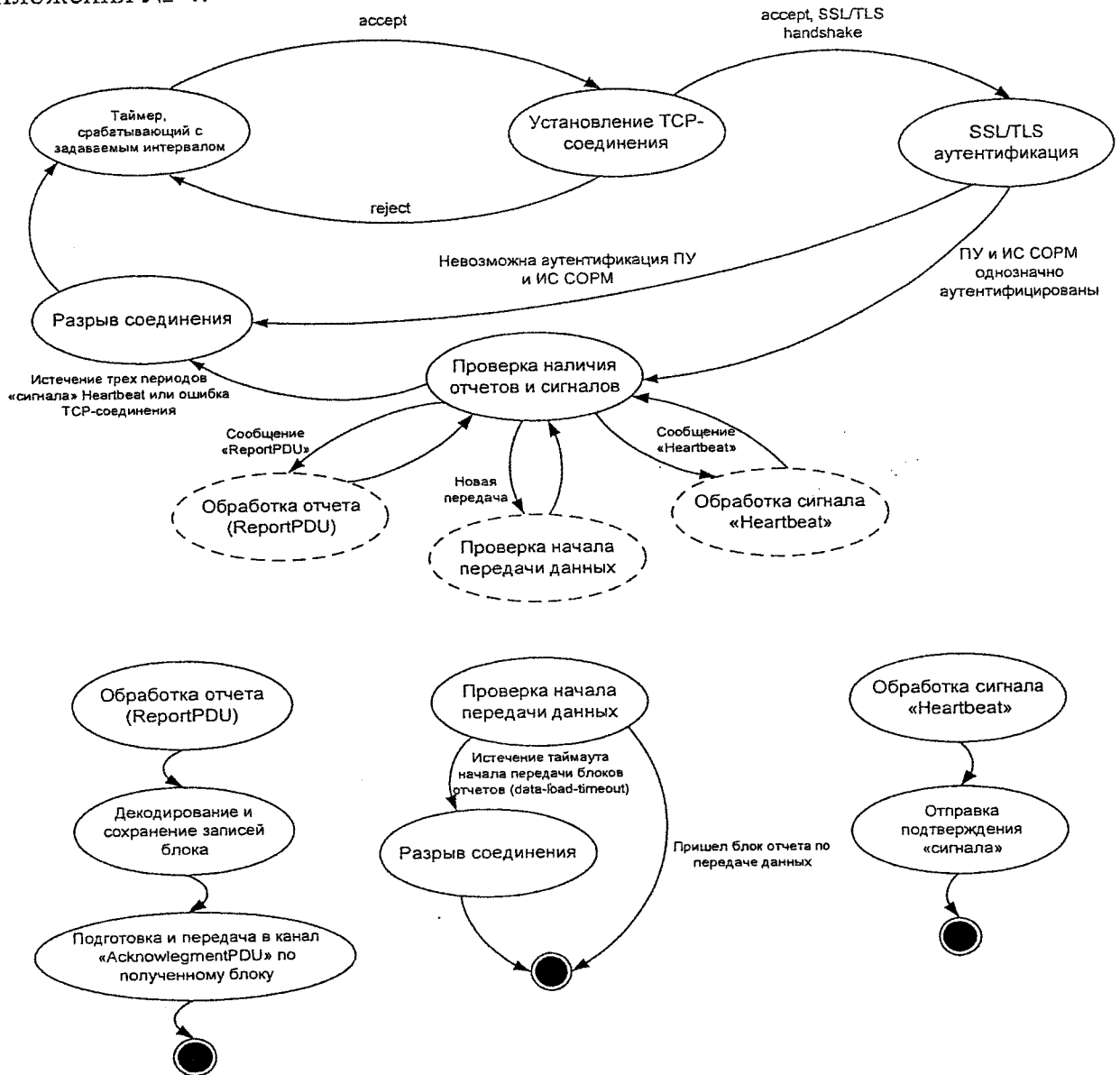
Рисунок 2. Диаграмма состояний перехода ПУ по кпд 2.
