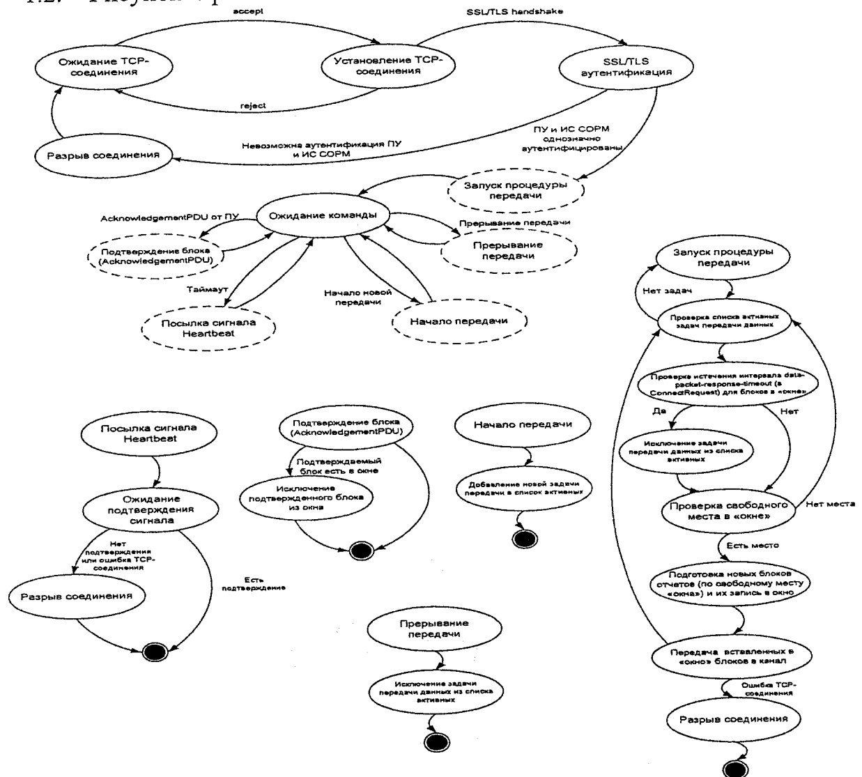
Рисунок 1. Диаграмма состояний перехода ТС ОРМ по кпд 2.
