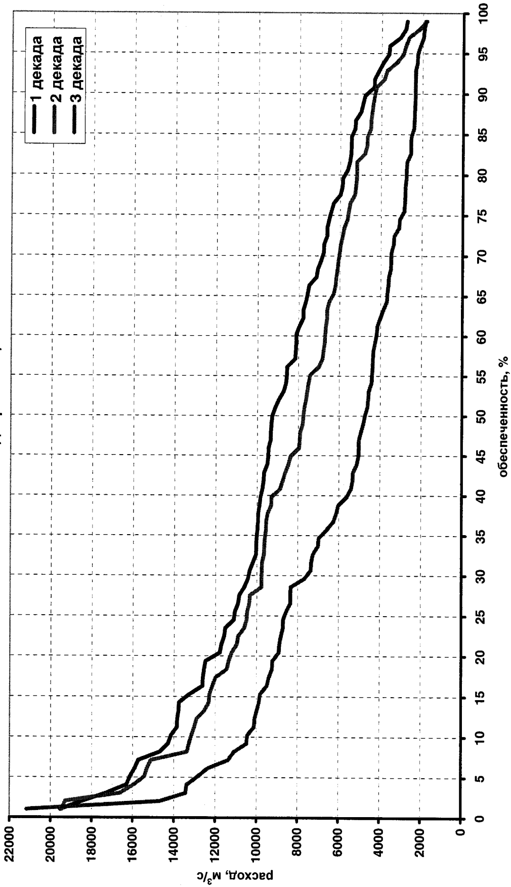
Расчетная обеспеченность среднедекадных расходов зарегулированного притока в Нижнекамское водохранилище в мае.
