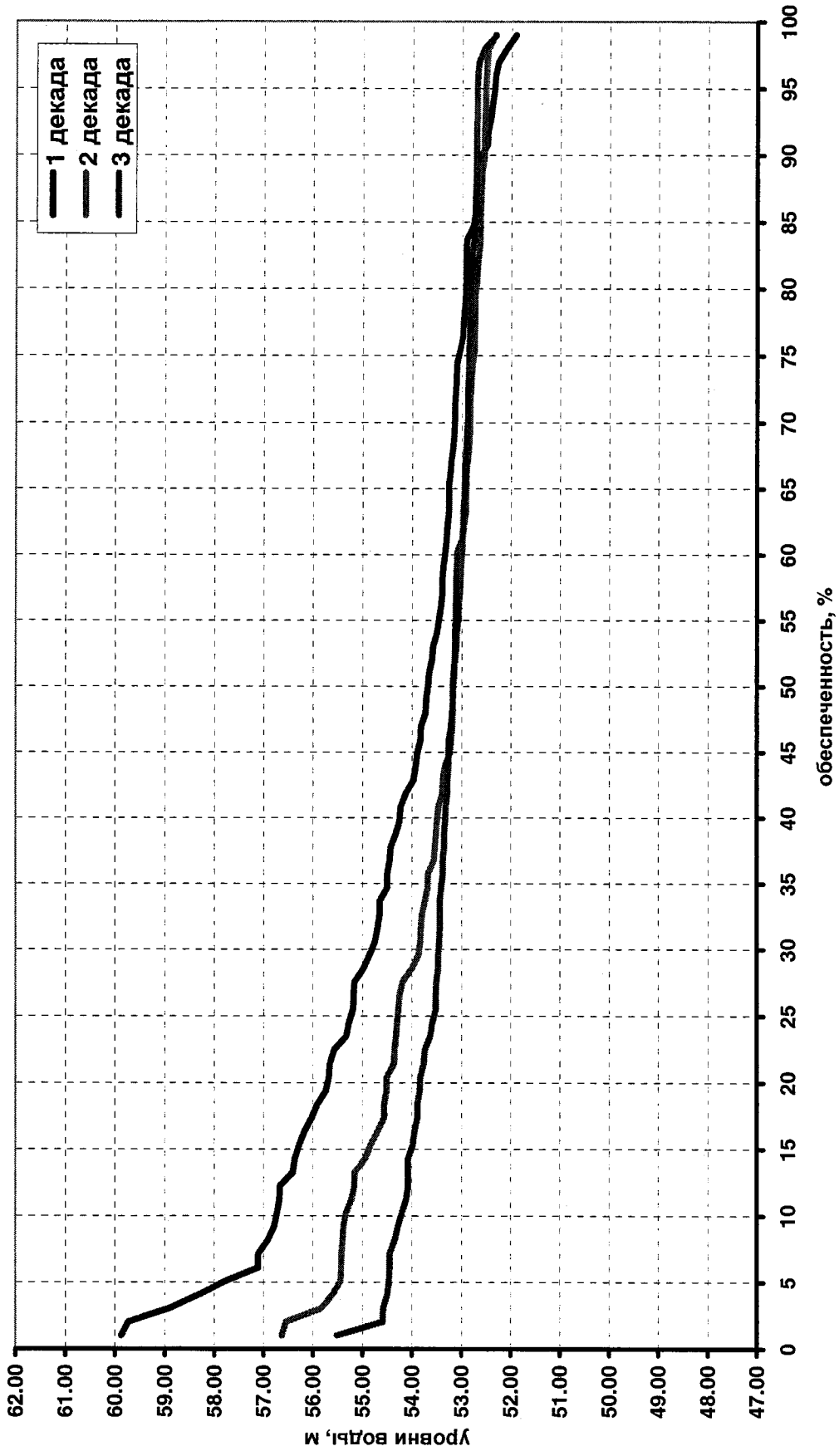
Расчетная обеспеченность уровнем воды в нижнем бьефе Нижнекамского ГУ в июне.
