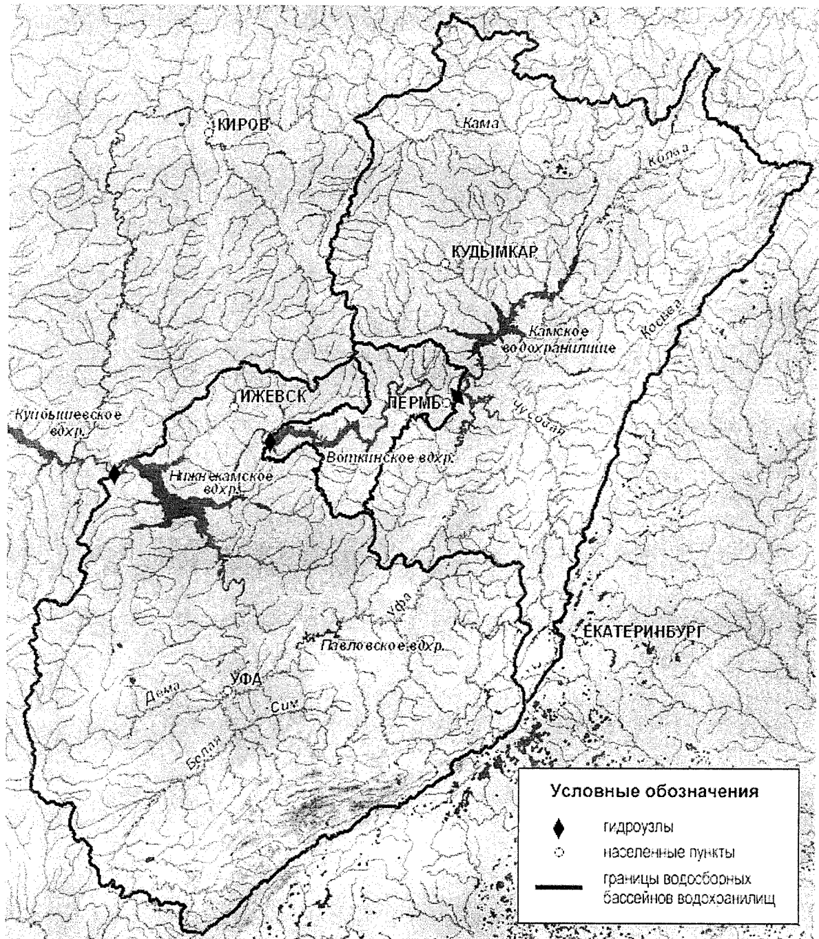
Схема каскада гидроузлов на р. Каме
